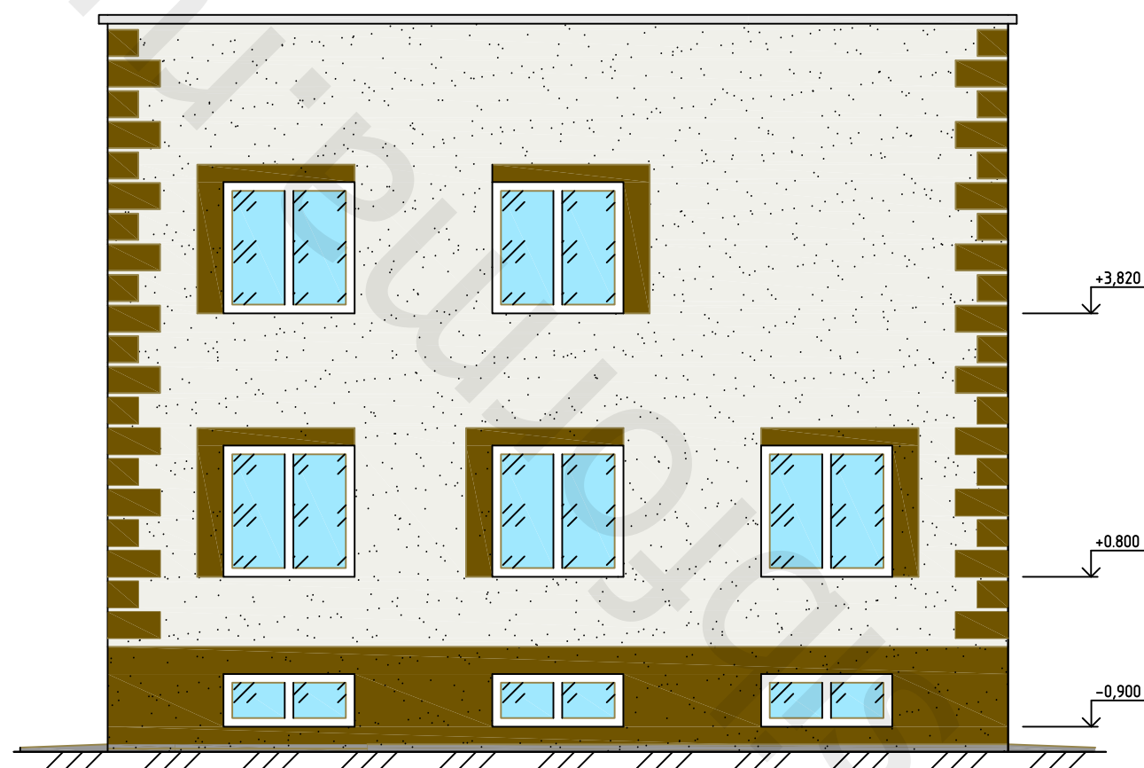
Восточный фасад
