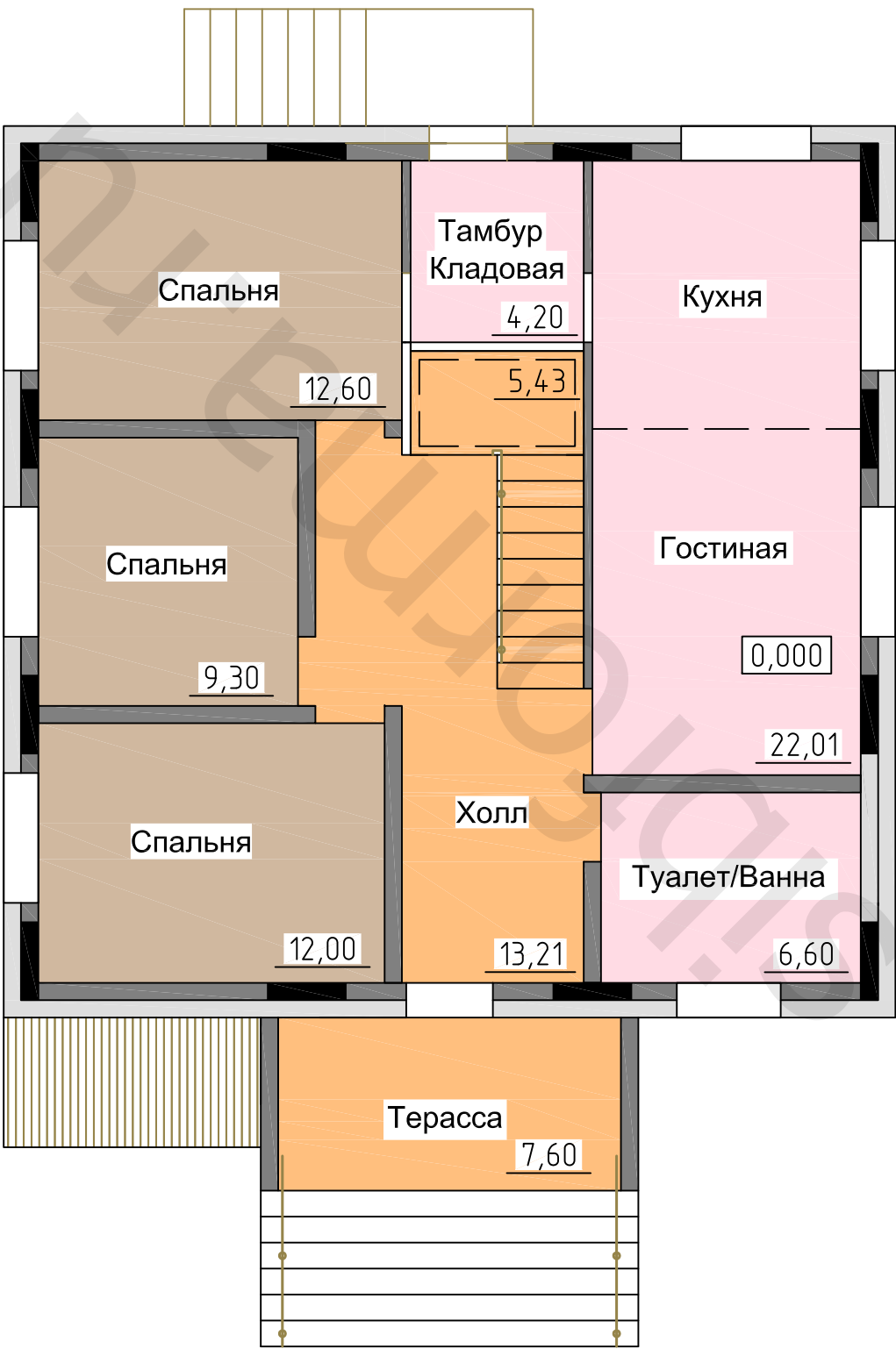
План 1 этажа
